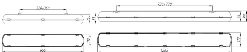
Рисунок 1. Габаритные размеры светильника ЛСП 2х18. Габаритные размеры светильника ЛСП 2х36.
